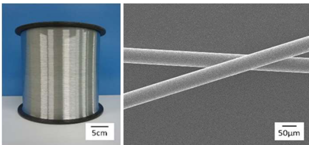
図1 アルミ鉄合金線 ポビン(φ80μm × 360km)
